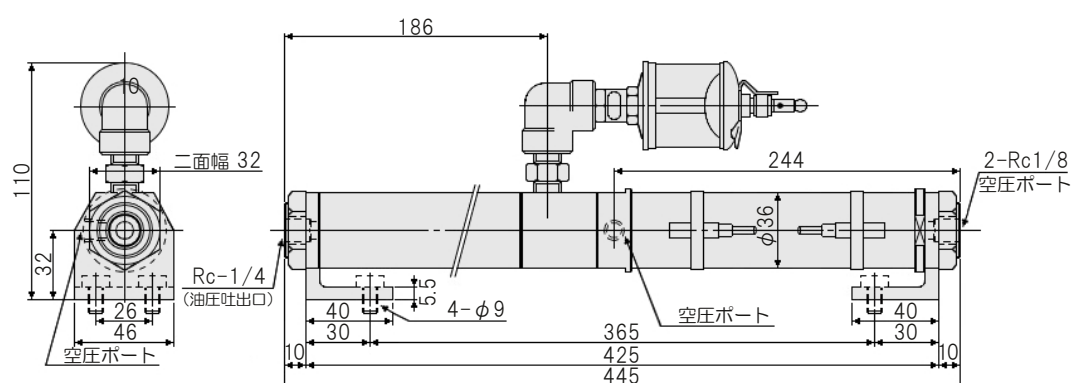
垂直取付
