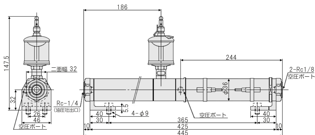
水平取付
